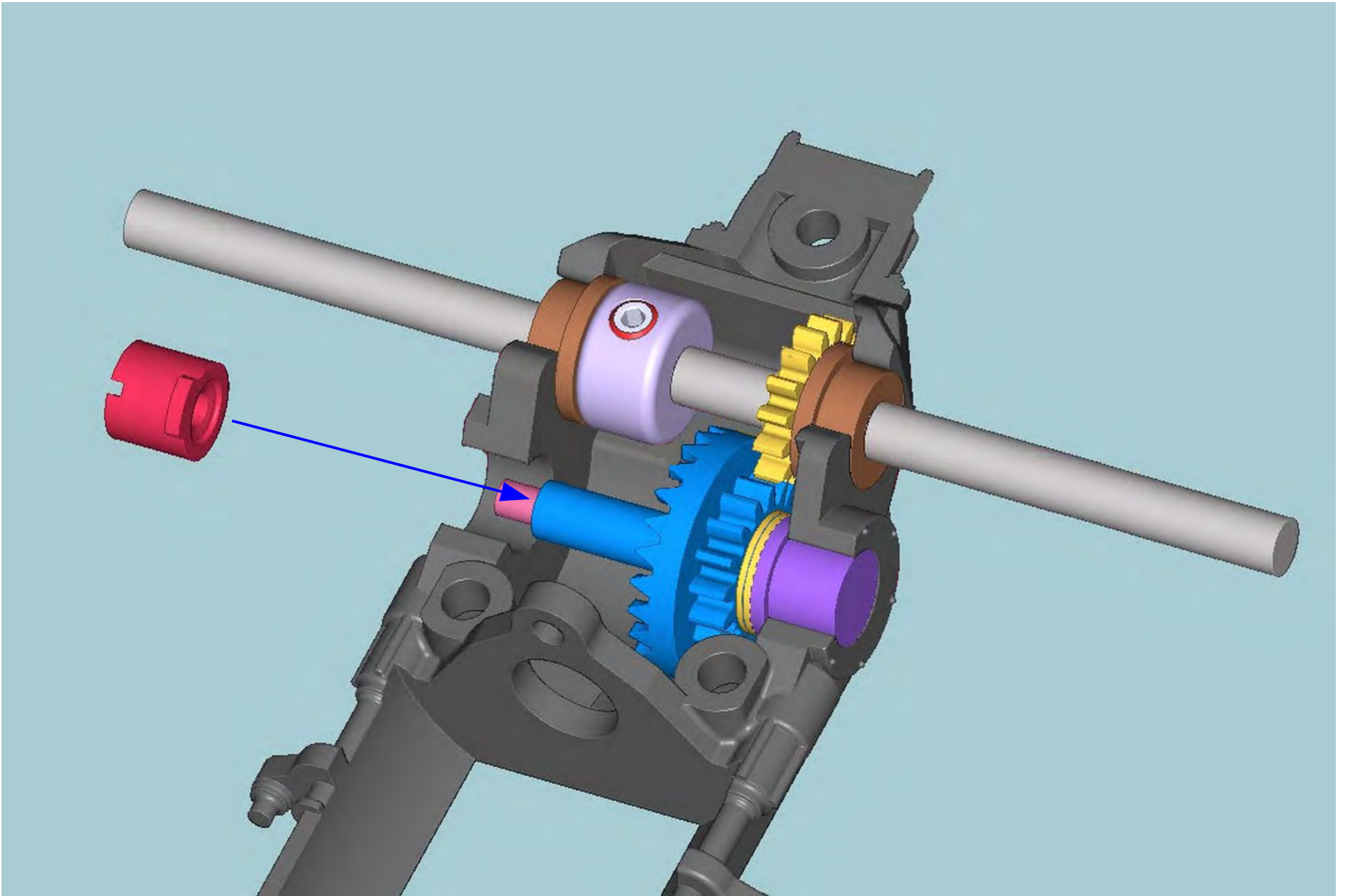
F1 motor mount assembly
