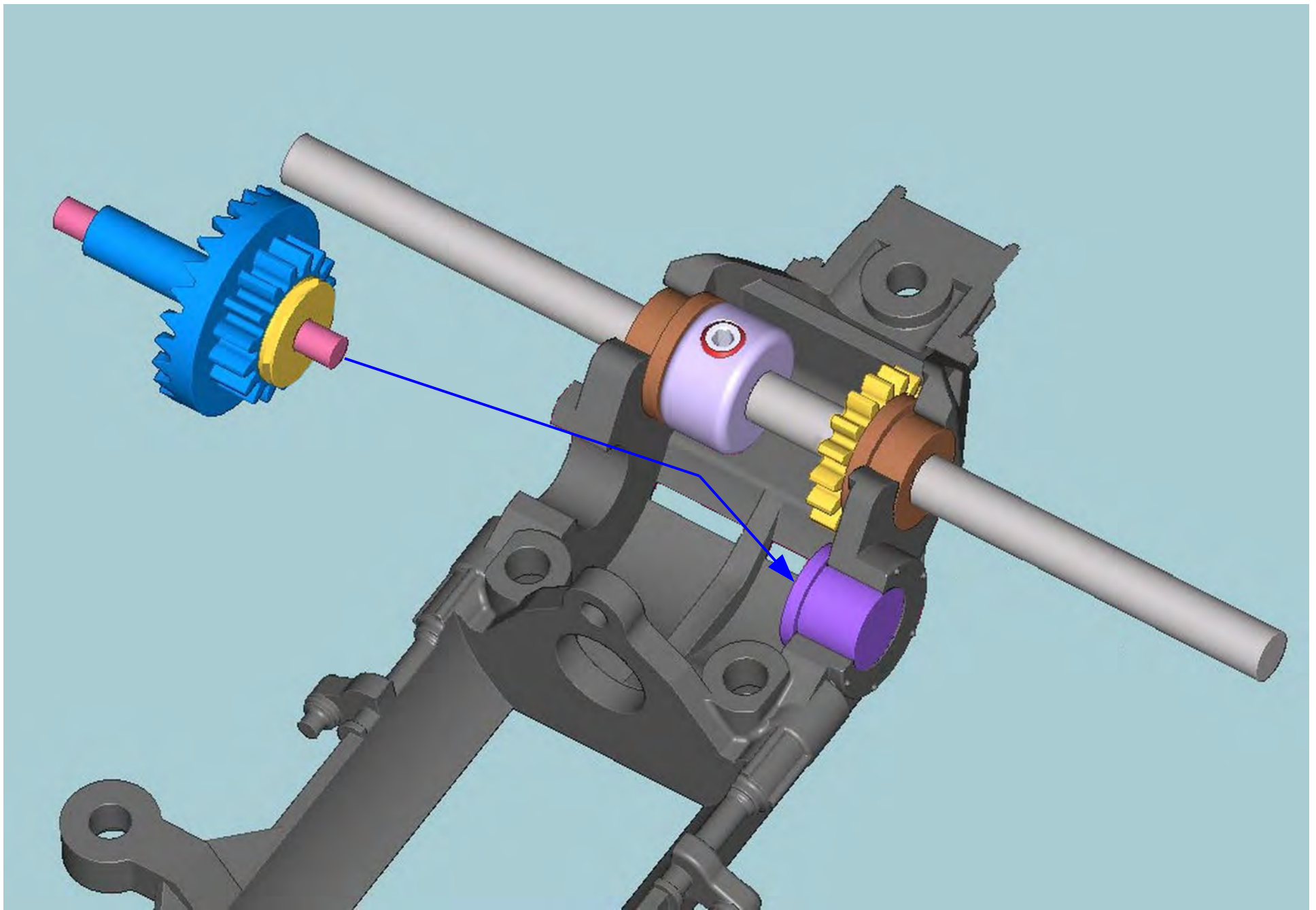
F1 motor mount assembly
